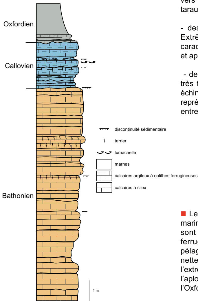
Coupe stratigraphique synthétique de la carrière de Mollets
